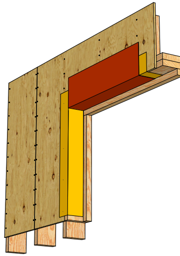
03. Metal trim
